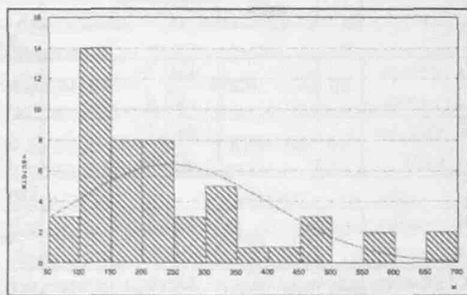
Рис. 1. Густота овражного расчленения на Корочанском (а) и Новооскольском (б) участках
