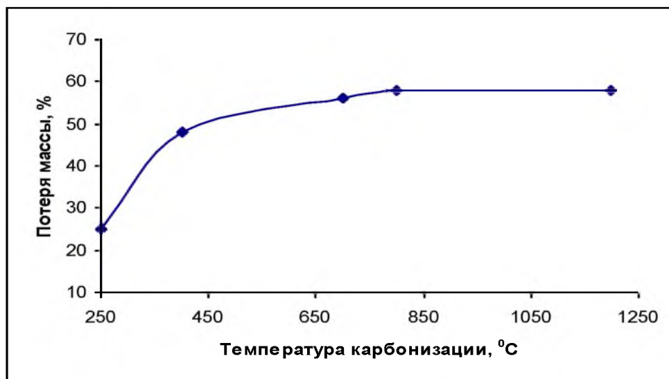
Рис. 1. Влияние температуры карбонизации на изменение массы скорлупы грецкого ореха Fig. 1. The influence of carbonization' temperature on change of mass of walnut shell
