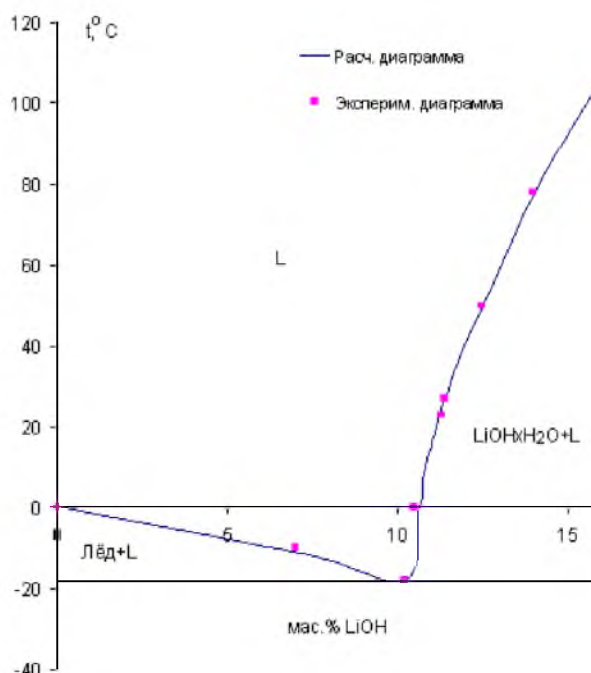
Рис. Экспериментальная и рассчитанная диаграммы состояния системы H_2O-LiOH Fig. Experimental and calculated phase diagrams of the system H_2O-LiOH
