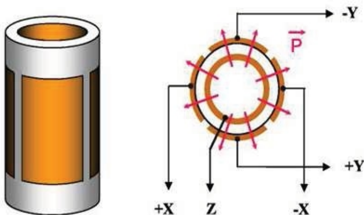
Рис. 2. Трубчатый пьезосканер [4].
