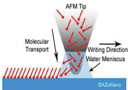
Рис. 1. Схематическая диаграмма, показывающая, как перьевая литография работает, на примере использования кантилевера атомно-силового микроскопа [3].
