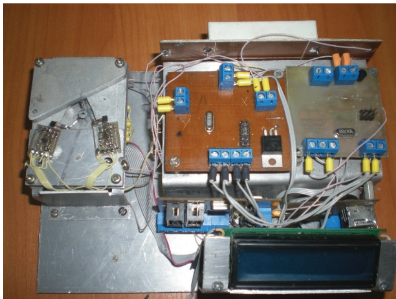
Рис. 10. Внешний вид макета устройства перьевой литографии.
