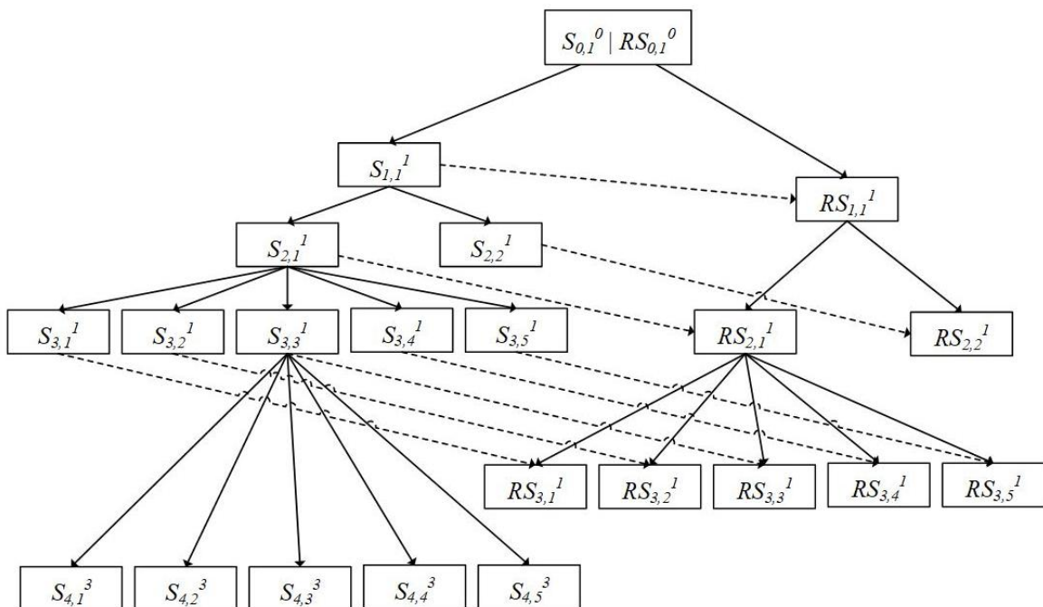
Рис. 4. Концептуальная схема предметной области «Автомобиль»
