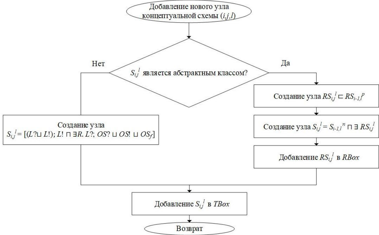
Рис. 3. Блок-схема подпрограммы добавления нового узла концептуальной системы
