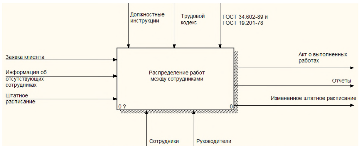
Рисунок 1 - Контекстная диаграмма
