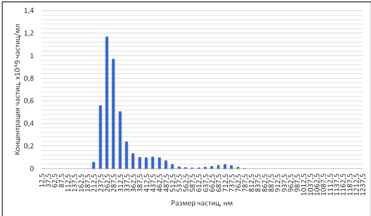
Рис. 8. Распределение частиц по размерам в образце нанокapsул спирулины в гуаровой камеди (соотношение ядро : оболочка 1 : 2) Fig. 8. Particle size distribution in a sample of spirulina nanocapsules in guar gum (core : shell ratio 1 : 2)
