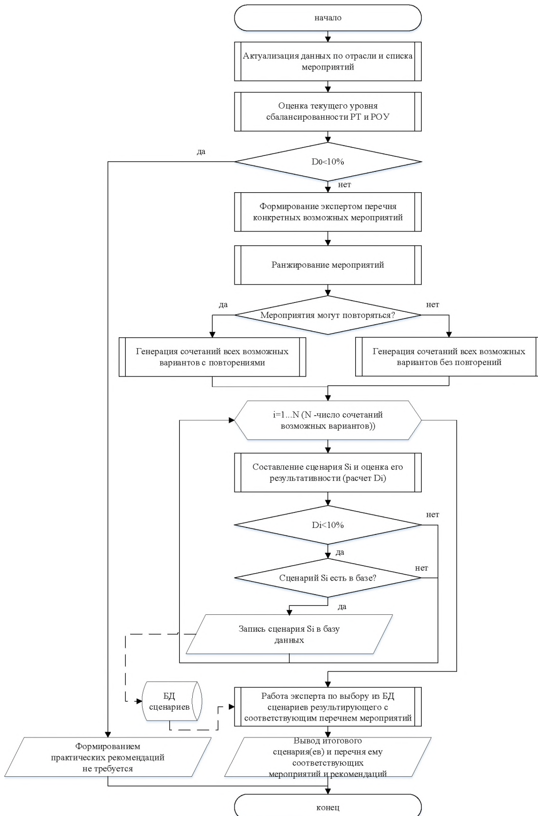
Рисунок 2 – Алгоритм формирования сценариев для РТ и РОУ
